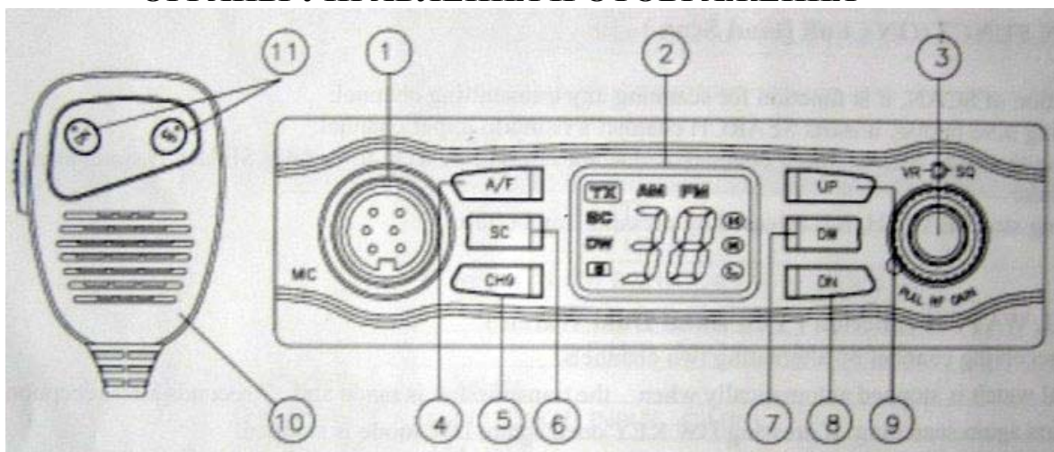
Рис. 1. Органы управления и отображения MJ-200Plus
